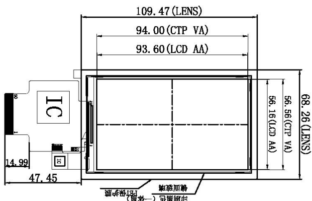
正视图
