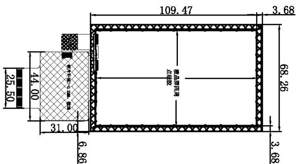
背视图
