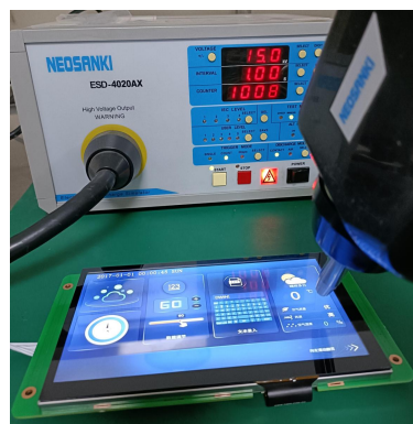
3.1 静电放电测试图
