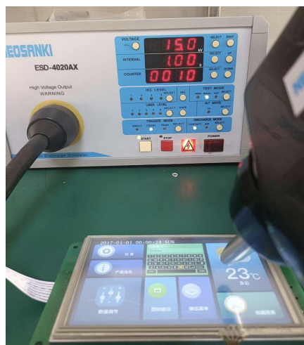
3.1 静电放电测试图
