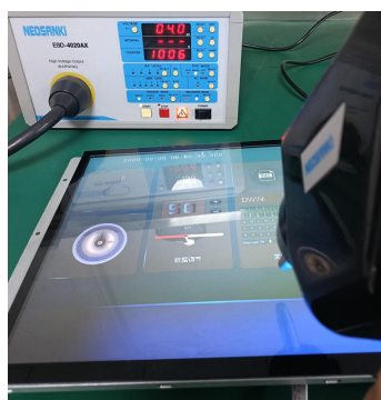
3.1 静电放电测试图
